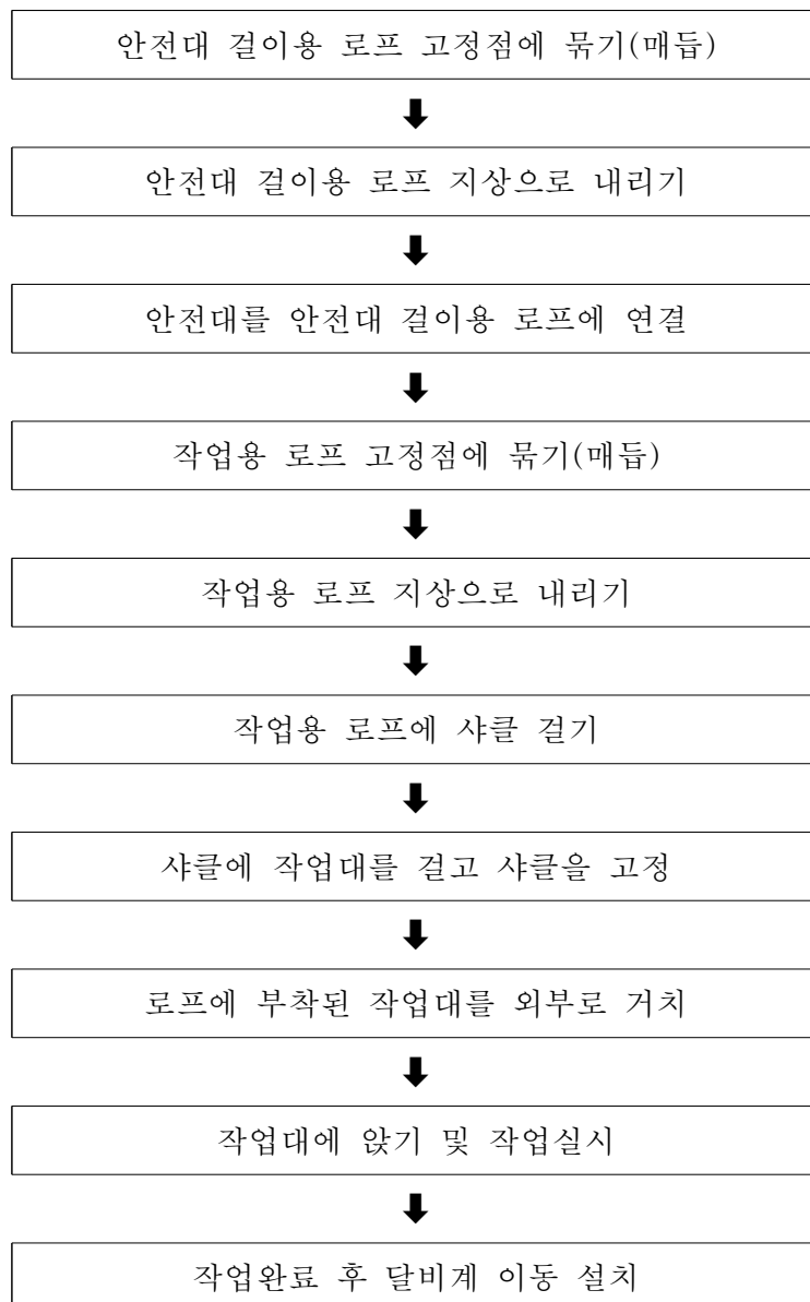
<그림 2> 달비계 작업순서
