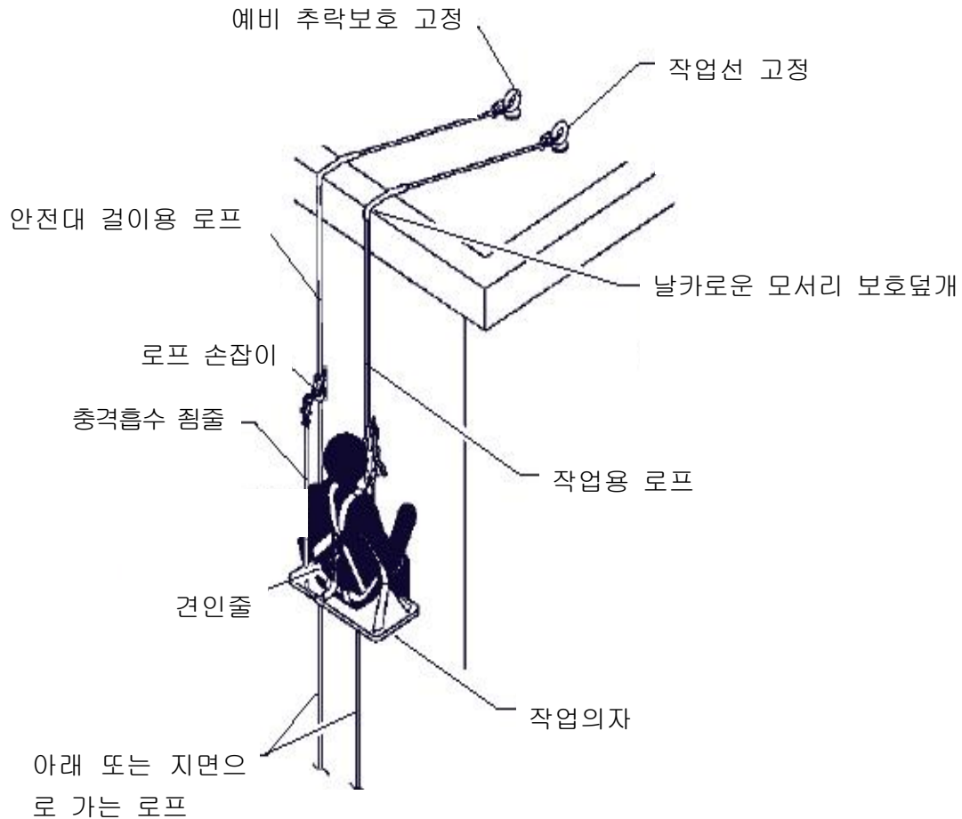
<그림 1> 달비계 구성요소
